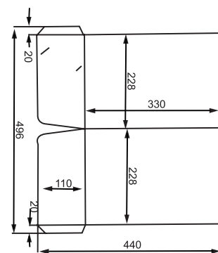
Платка 9 330x228 Склеивка
