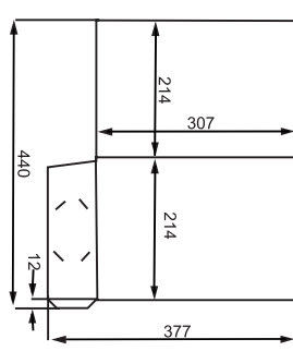
Платка 10 302x214 Склеивка
