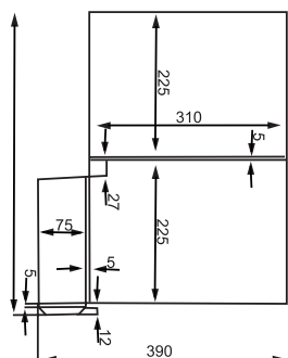
Платка 4 310x225 Толщ. 5 Склеивка
