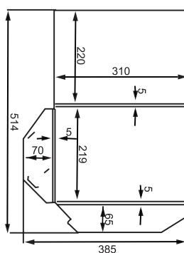
Платка 14 303x220 Толщ. 5 Замок
