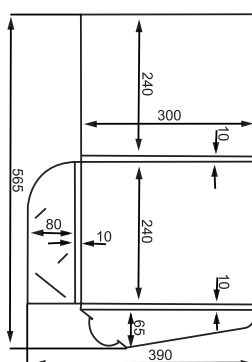
Платка 6 300x240 Толщ. 10 Замок
