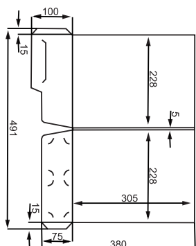
Платка 3 305x228 Толщ. 5 Склеивка
