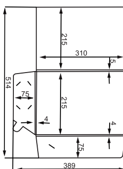
Платка 7 310x215 Толщ. 5 Замок
