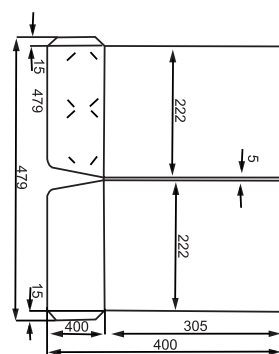
Платка 1 305x222 Толщ. 5 Склеивка
