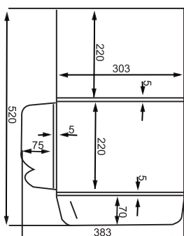
Платка 11 303x220 Толщ. 5 Замок
