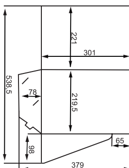
Платка 12 303x220 Замок
