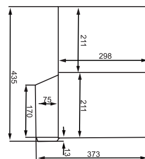
Платка 13 302x14 Склеивка
